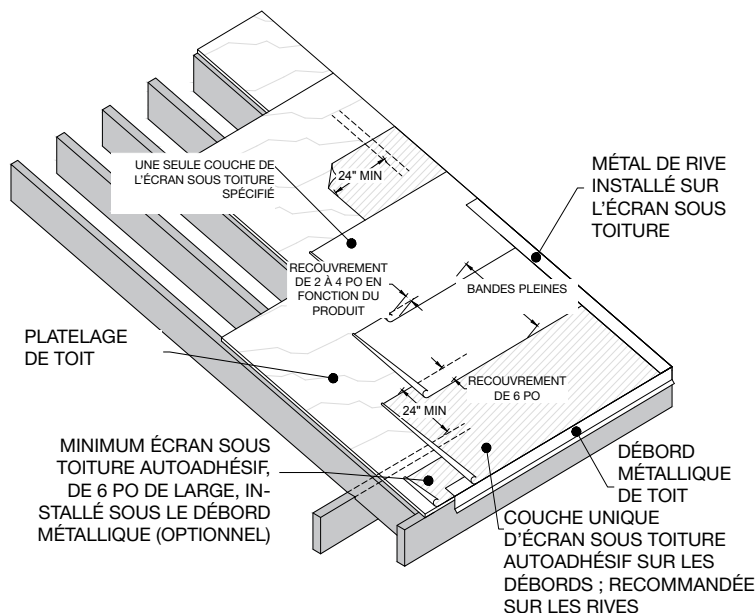
Figure 3 – Application des couches de finition autoadhésives pour des pentes de toit supérieures ou égales à 4:12 (régions avec accumulation de glace)
