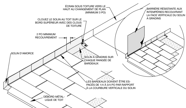
Figure 12 – Pose de solins à gradins au niveau des transitions toiture/paroi verticale
