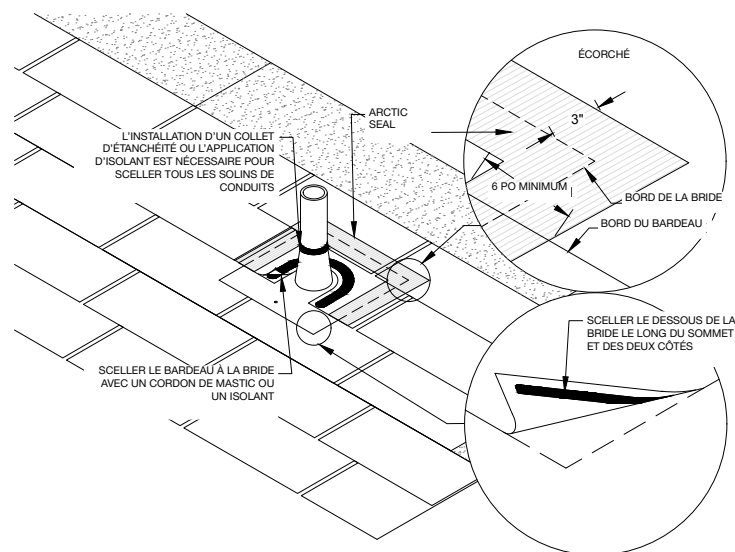
Figure 13 – Pose de solins de conduits d'évent
