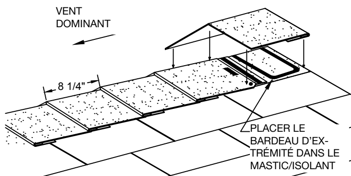
Figure 26 – Variante pour le positionnement et la fixation de l'embout EZ-Ridge™
