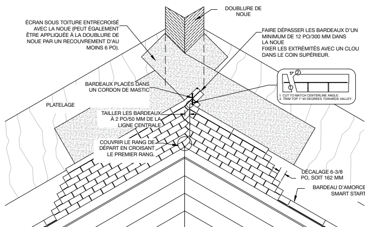
Figure 10 – Pose de noues à double tranchis
