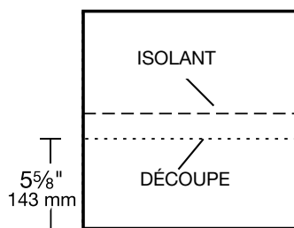
Figure 18 – Bande de bardeaux RidgeFlex™ pour en faire un bardeau d'amorce d'arête et de faîtage
