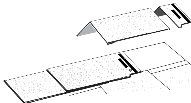
Figure 25 – Découpe d'un bardeau EZ-Ridge™ en embout
