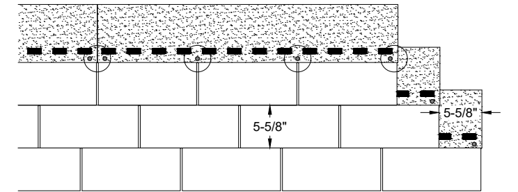
Figure 6 – Modèle de fixation à 3 onglets et 4 clous
