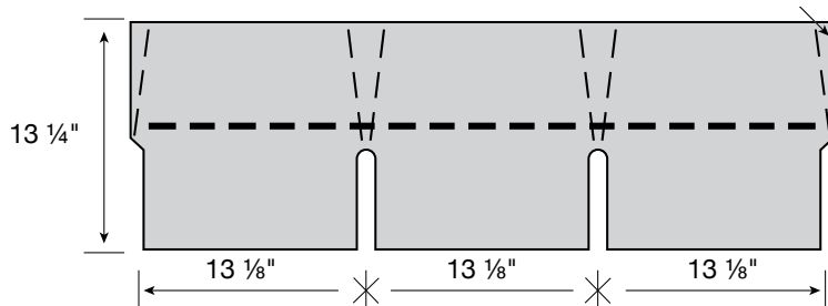
Figure 22 – Découpe d'un bardeau à 3 jupes Dura-Seal™ AR pour en faire des bardeaux de faîtage et d'arête
