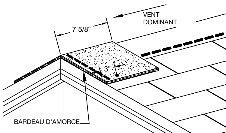
Figure 19 – Positionnement et fixation du bardeau d'amorce RidgeFlex™
