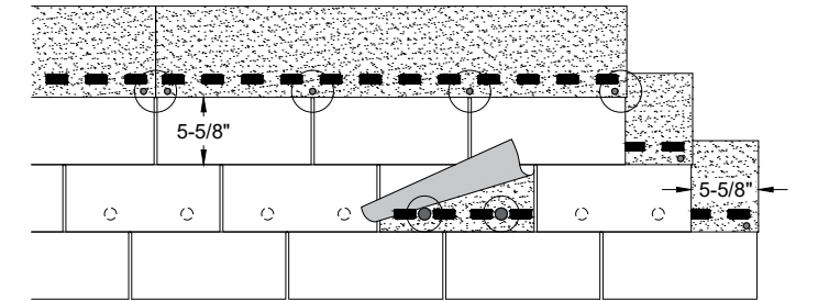
Figure 7 – Collage à la main de bardeaux à 3 jupes
