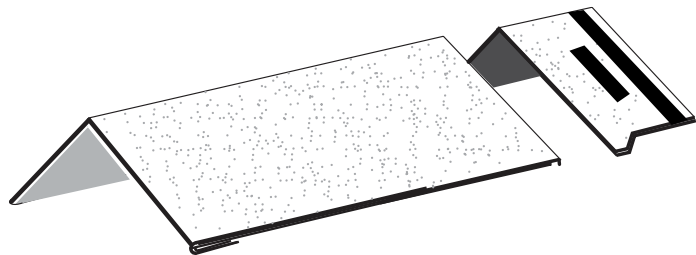
Figure 23 – Découpe d'un bardeau EZ-Ridge™ pour en faire un bardeau d'amorce d'arête et de faitage
