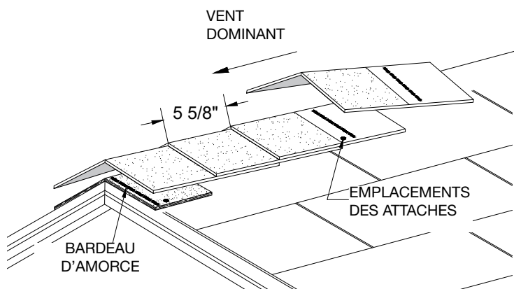
Figure 20 – Positionnement et fixation des bardeaux RidgeFlex™, en conservant un pureau de 5-58 po
