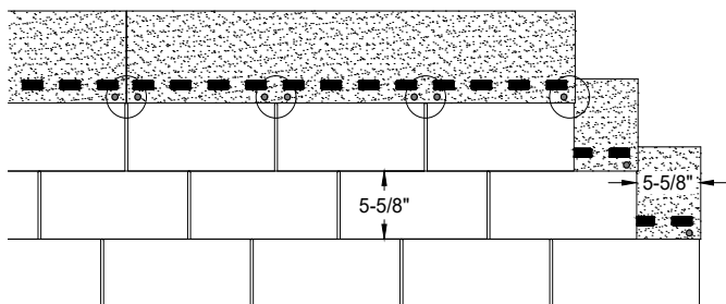
Figure 8 – Modèle de fixation à 3 onglets et 6 clous
