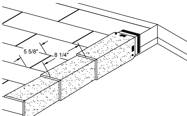
Figure 27 – Pose des bardeaux EZ-Ridge™ sur les rives de toit
