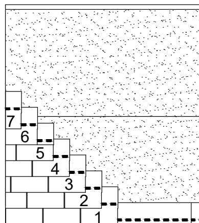
Figure 9 – Disposition des bardeaux à 3 jupes
