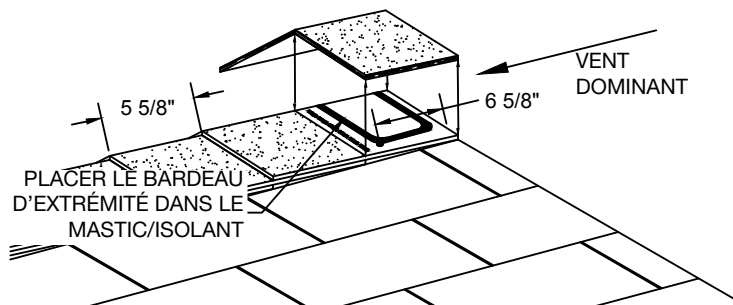
Figure 21 – Pose des bardeaux de la gamme RidgeFlex™ ; Embout fixé dans le mastic
