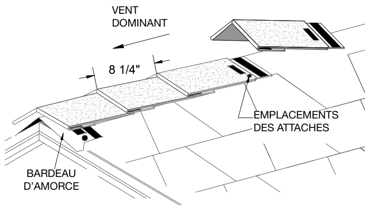
Figure 24 – Positionnement et fixation des bardeaux EZ-Ridge™, afin de conserver un pureau de 8¼ po
