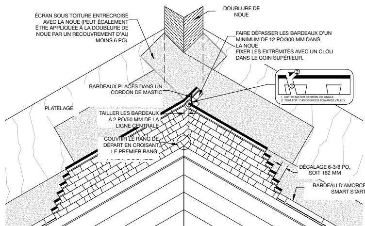
Figure 11 – Pose de noues à double tranchis
