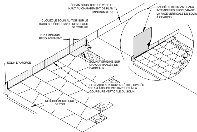
Figure 13 – Pose de solins à gradins au niveau des transitions toiture/paroi verticale
