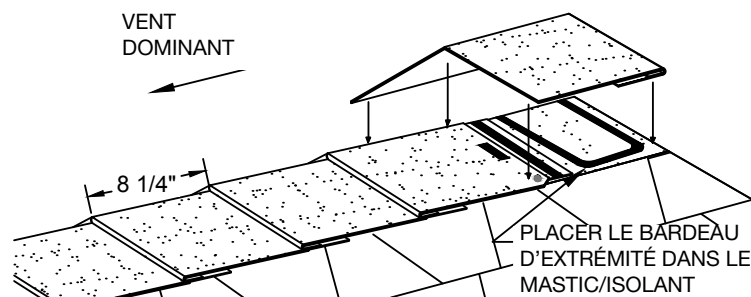
Figure 26 – Variante pour le positionnement et la fixation de l'embout EZ-Ridge™
