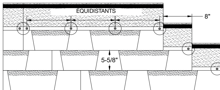
Figure 6 – Plan de clouage 4 clous, lamellés
