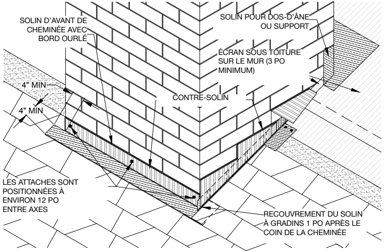
Figure 15 – Contre-solin et allège de cheminée
