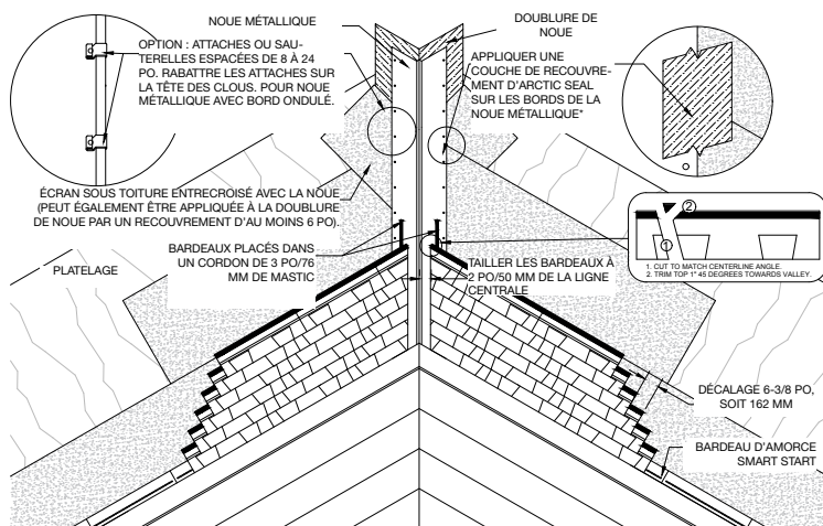
Figure 12 – Pose de noues en métal ouvertes
