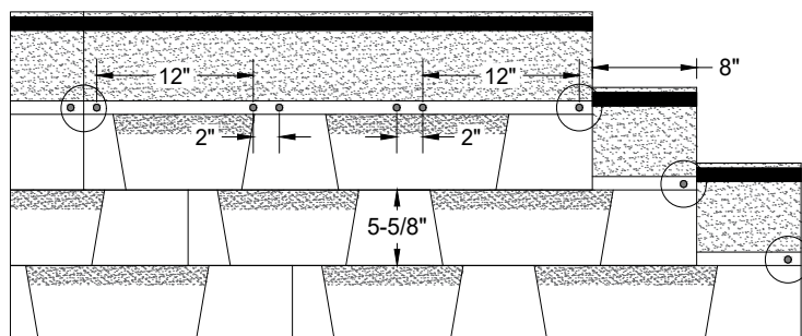
Figure 9 – Plan de clouage alternatif 6 clous, bardeaux lamellés
