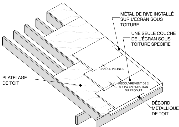
Figure 1 – Application de la couche de finition pour des pentes de toit supérieures ou égales à 4:12 (régions exemptes d'accumulation de glace)
