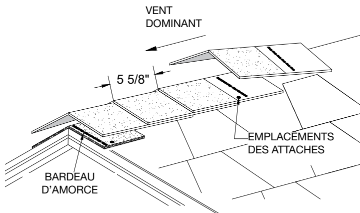
Figure 21 – Positionnement et fixation des bardeaux RidgeFlex™, en conservant un pureau de 5-58 po
