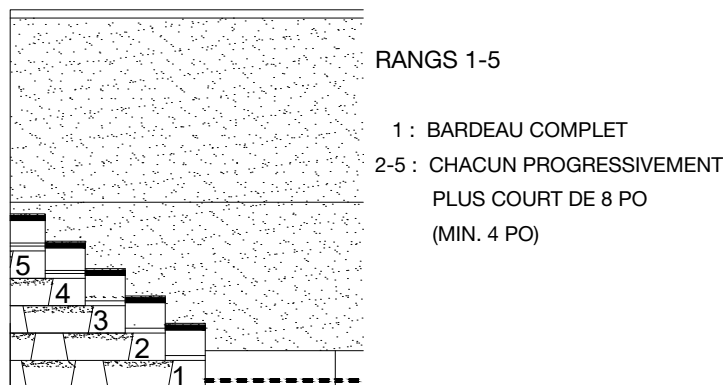
Figure 10 – Disposition des bardeaux lamellés
