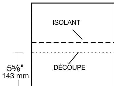
Figure 19 – Bande de bardeaux de faîtage RidgeFlex™ pour en faire un bardeau d'amorce d'arête et de faîtage
