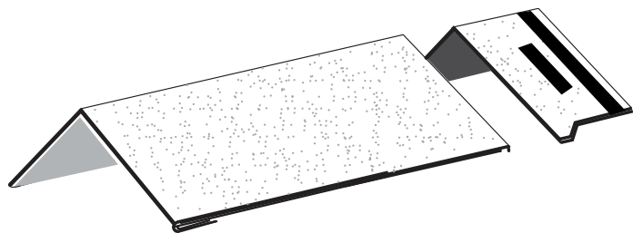
Figure 23 – Découpe d'un bardeau EZ-Ridge™ pour en faire un bardeau d'amorce d'arête et de faîtage
