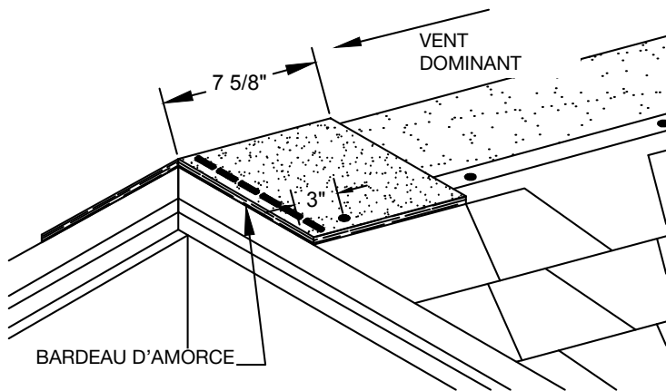
Figure 20 – Positionnement et fixation du bardeau d'amorce RidgeFlex™ Bardeau d'amorce
