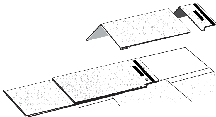
Figure 25 – Découpe d'un bardeau EZ-Ridge™ en embout
