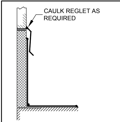
OPTION: CUT-IN REGLET
