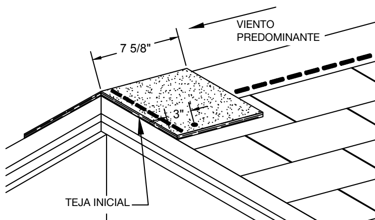
Figura 19 - Emplazamiento y sujeción de la teja inicial RidgeFlex™
