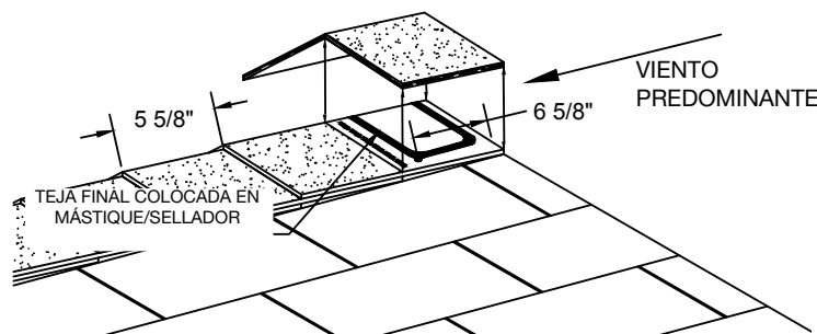
Figura 21 - Instalación de las tejas RidgeFlex™; tapa extrema colocada en mástique
