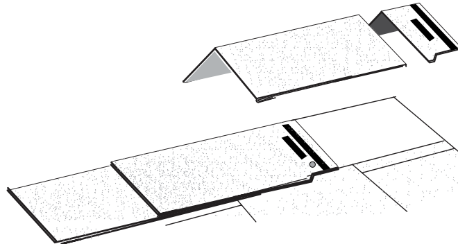
Figura 25 - Teja EZ-Ridge™ cortada para crear una tapa extrema
