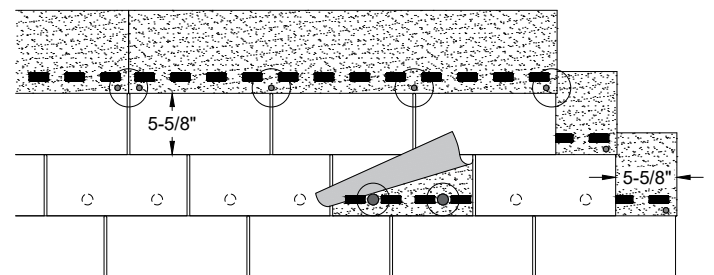
Figura 7 - Sellado manual de tejas de 3 pestañas
