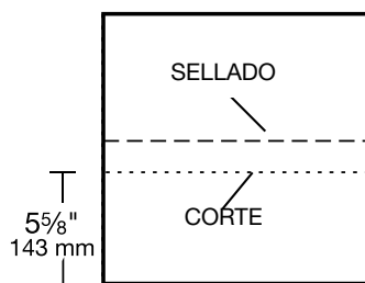
Figura 18 - Tira de tejas RidgeFlex™ para su empleo como teja inicial para limatesas y cumbresas
