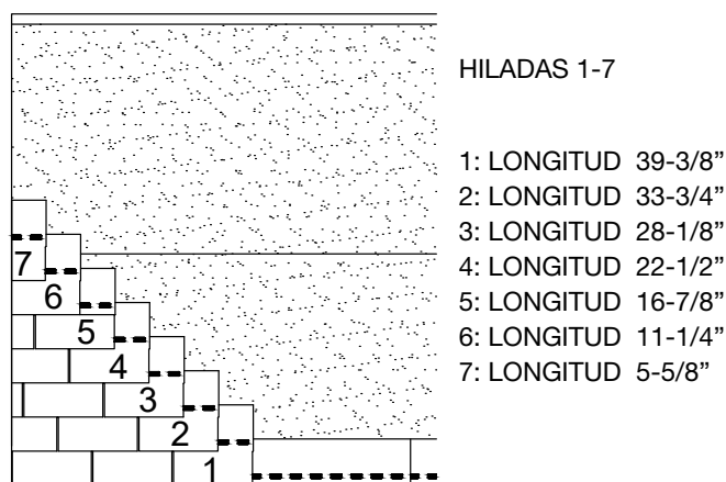
Figura 9 - Patrón de disposición de tejas de 3 pestañas
