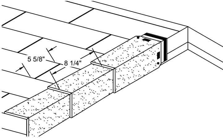
Figura 27 - Instalación de las tejas EZ-Ridge™ en los bordes de faldón del techo
