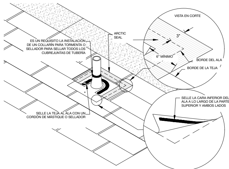
Figura 13 - Aplicación de cubrejuntas de tubería de ventilación
