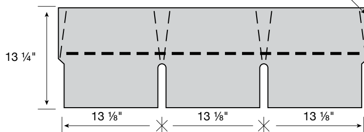
Figura 22 - Corte de una teja de 3 pestañas Dura-Seal™ AR para su empleo como teja para limatesas y cumbresas
