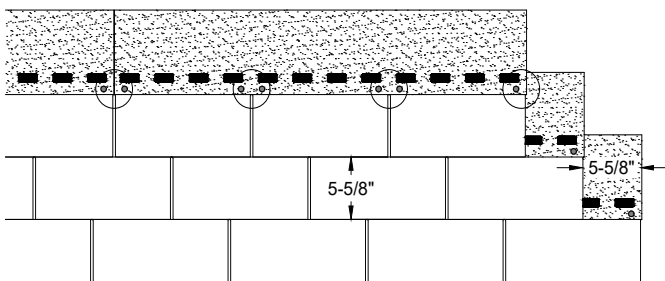
Figura 8 - Patrón de sujeción de 6 clavos para tejas de 3 pestañas
