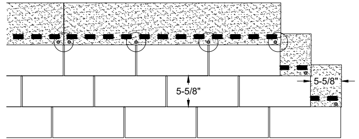
Figura 6 - Patrón de sujeción de 4 clavos para tejas de 3 pestañas
