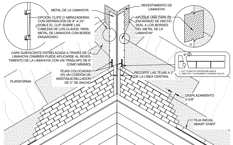
Figura 11 - Aplicación en limahoya metálica abierta
