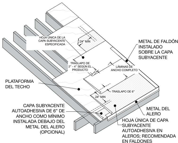
Figura 3 - Aplicación de capas subyacentes de techo y autoadhesivas en techos de pendiente 4:12 y mayores (regiones con rebordes de hielo)
