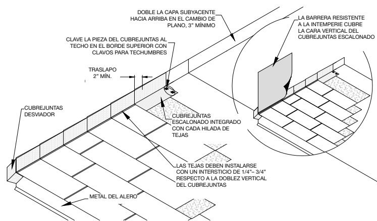
Figura 12 - Aplicación de cubrejuntas escalonado en transiciones techo-pared lateral
