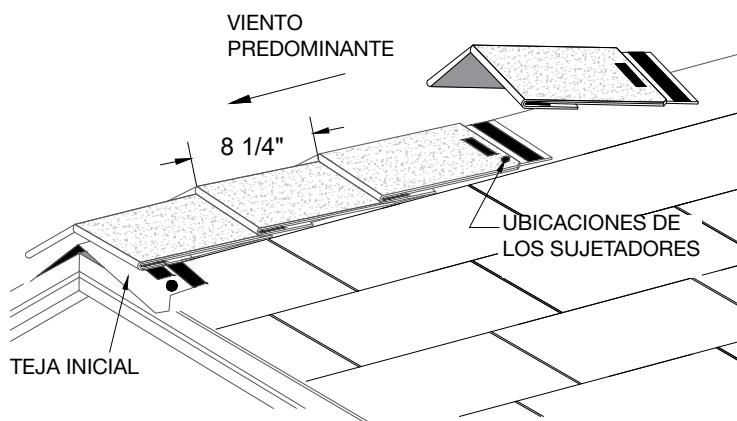
Figura 24 - Emplazamiento y sujeción de las tejas EZ-Ridge™, manteniendo la exposición de 8- \frac{1}{4} "
