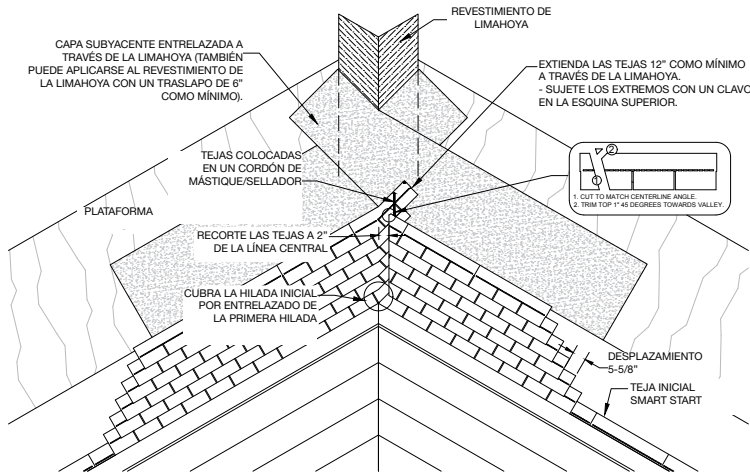
Figura 10 - Aplicación en limahoya cerrada
