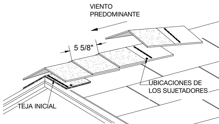
Figura 20 - Emplazamiento y sujeción de las tejas RidgeFlex™, manteniendo la exposición de 5\frac{5}{8} "
