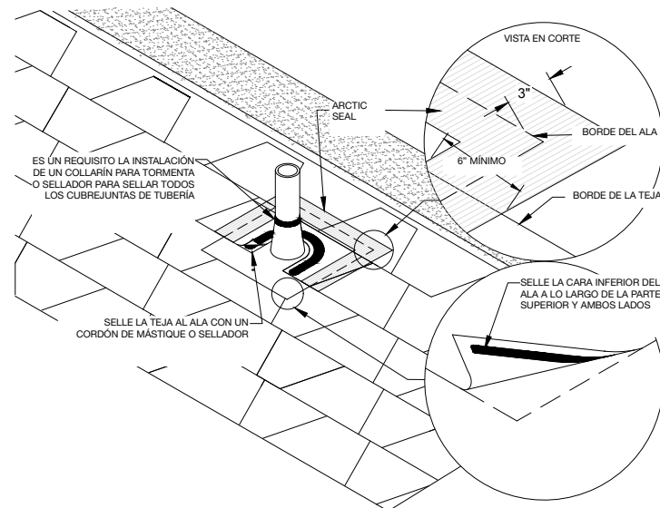
Figura 14 - Aplicación de cubrejuntas de tubería de ventilación
