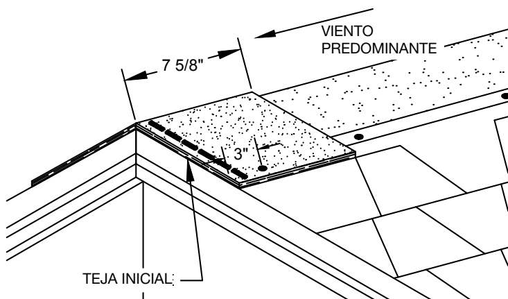
Figura 20 - Emplazamiento y sujeción de la teja inicial RidgeFlex™
