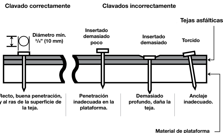
Figura 5 - Instrucciones de clavado
