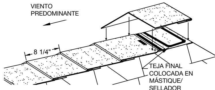
Figura 26 - Posicionamiento y sujeción opcional de la tapa extrema EZ-Ridge™
