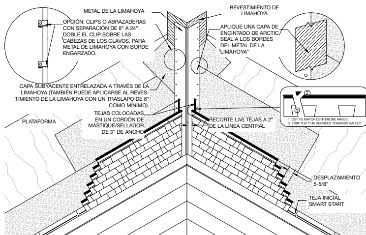
Figura 12 - Aplicación en limahoya metálica abierta
