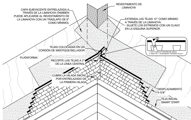
Figura 11 - Aplicación en limahoya cerrada
