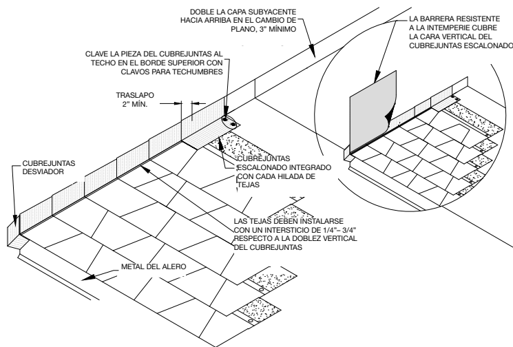
Figura 13 - Aplicación de cubrejuntas escalonado en transiciones techo-pared lateral
