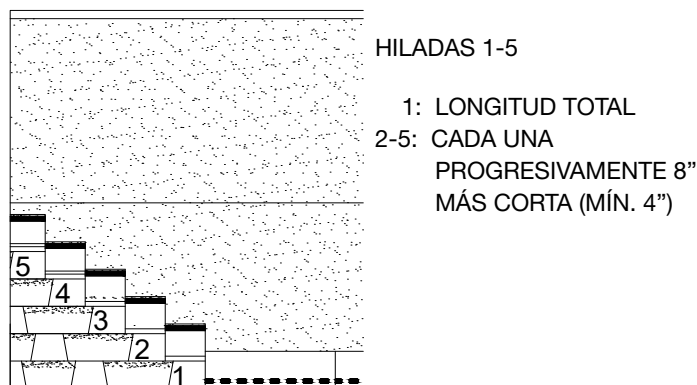
Figura 10 - Patrón de disposición de tejas laminadas
