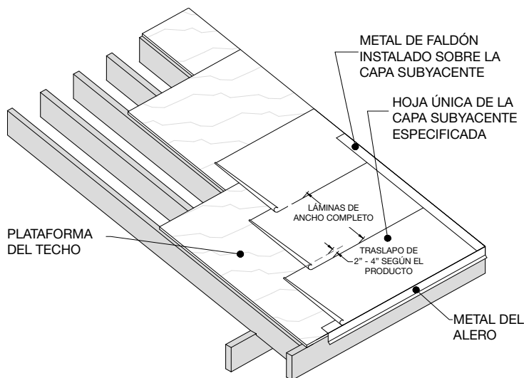
Figura 1 - Aplicación de capa subyacente de techo en techos de pendiente 4:12 y mayores (regiones sin rebordes de hielo)
