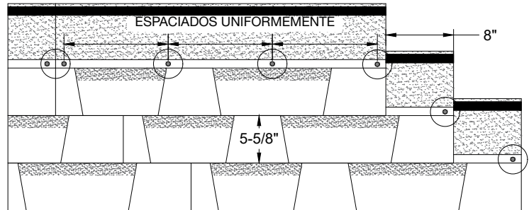
Figura 6 - Patrón de sujeción de 4 clavos para tejas laminadas
