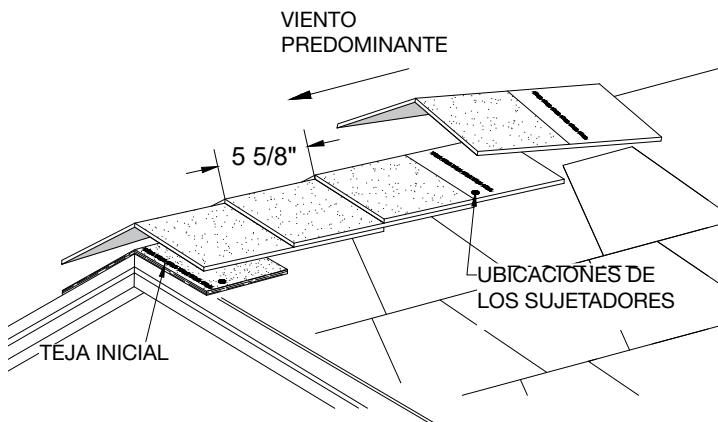
Figura 21 - Emplazamiento y sujeción de las tejas RidgeFlex™, manteniendo la exposición de 5- \frac{5}{8} "
