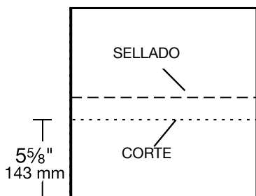
Figura 19 - Tira de tejas RidgeFlex™ para su empleo como teja inicial en limatesas y cumbres
