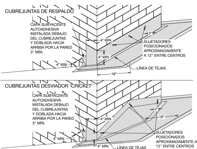
Figura 16 - Aplicaciones de cubrejuntas de caballetes y desviadores 'crickets' de chimenea
