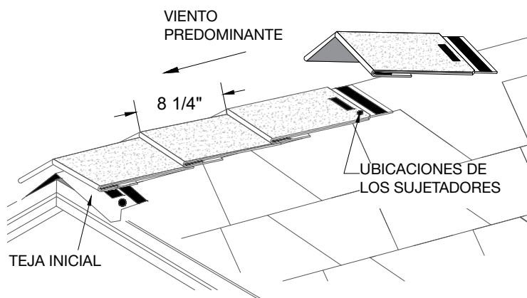
Figura 24 - Emplazamiento y sujeción de las tejas EZ-Ridge™,
