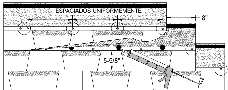
Figura 7 - Sellado manual de tejas laminadas
