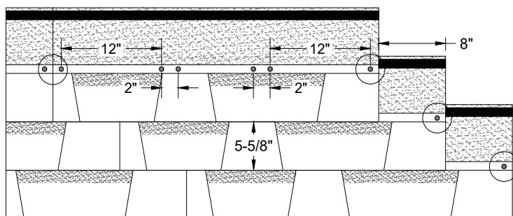
Figura 9 - Patrón de sujeción alternativo de 6 clavos para tejas laminadas
