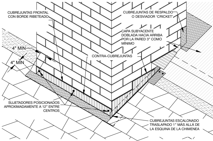
Figura 15 - Aplicaciones de contra-cubrejuntas y placa delantal de chimenea
